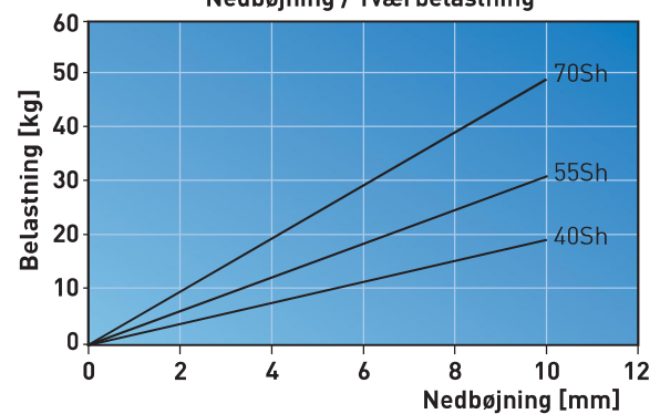
Nedbøjning / Tværbelastning
